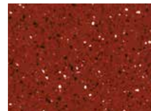
jaspis 4094
