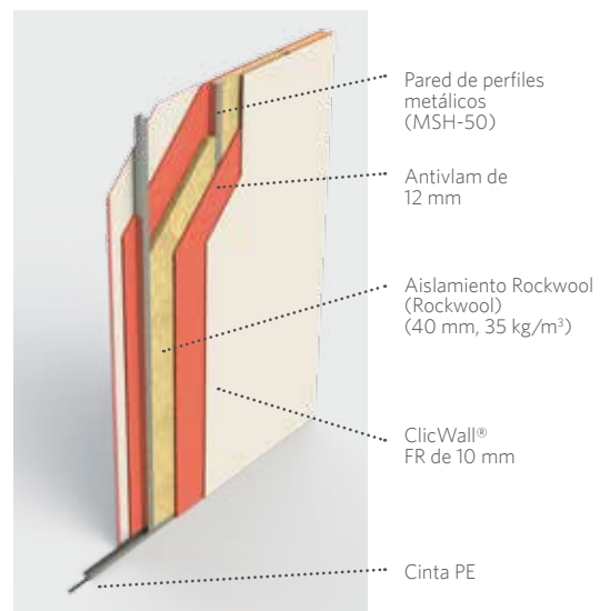
Antivlam fijado a pared de perfiles metálicos: tornillos para madera de 4,0 x 25 ClicWall® FR sobre Antivlam: unión con polímero MS
