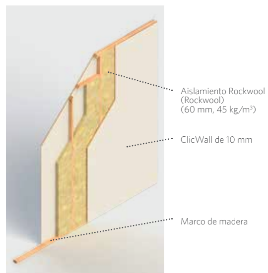
ClicWall fijado a listones de madera: tornillos para madera de 3,5 x 16
