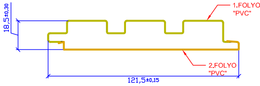
PVC FOLYO FREZELENMİŞ GÖRÜNÜM MILLED PVC FOIL VIEW
